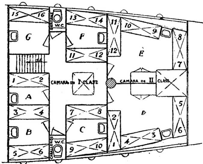
CUBIERTA PRIMERA
