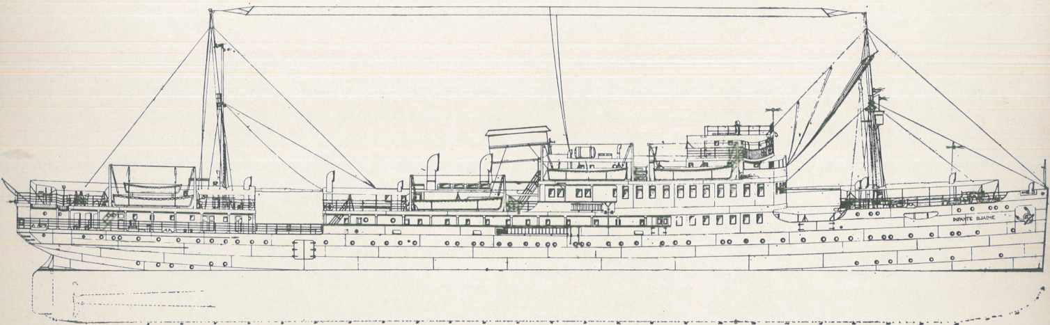
PLANOS GENERALES
